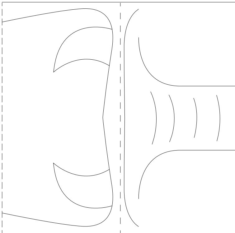
Patron de la marionnette à main dragon : la gueule et le cou (à agrandir à 140 %)
